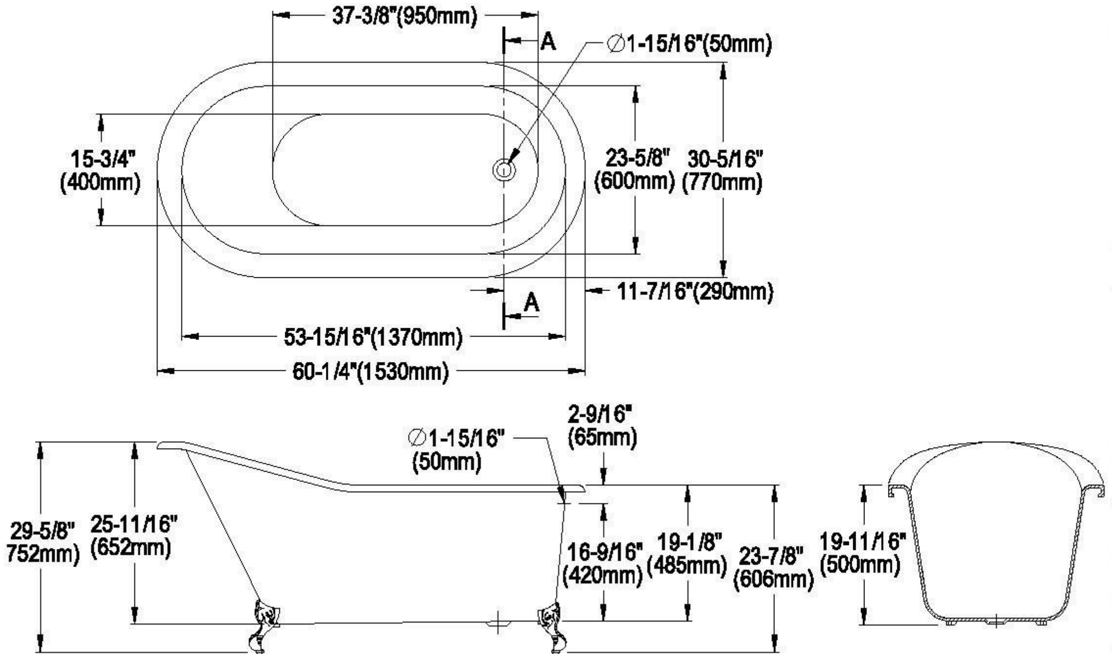
Section A-A
